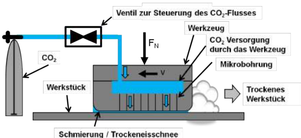
Fig. 3: Prinzipsskizze des Versuchsaufbaus zur Aufnahme der Rückhaltekräfte im Modellversuch Streifenziehen
