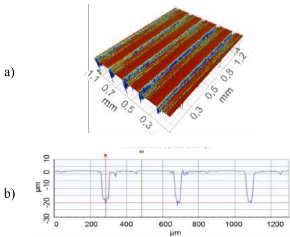
Fig. 15: a) Bild einer linienstrukturierten Oberfläche aus einer interferometrischen Messung und b) der entsprechende Querschnitt dieser Oberfläche.
