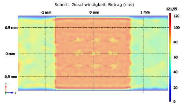
Fig. 25: Darstellung der Geschwindigkeit von \text{CO}_2 auf Höhe der sich bewegten Werkstückoberfläche.
