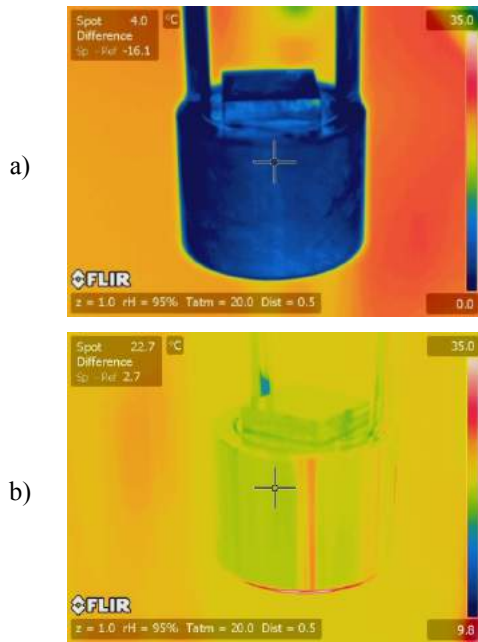
Fig. 18: Aufnahmen einer IR-Kamera des Probenstüchs. a) Gleichmäßige Verteilung der Temperatur bei abgeschaltetem Thermostat, b) mit eingeschaltetem Thermostat stellt sich nach 15 min eine gleichmäßige Temperatur von 4 °C ein.
