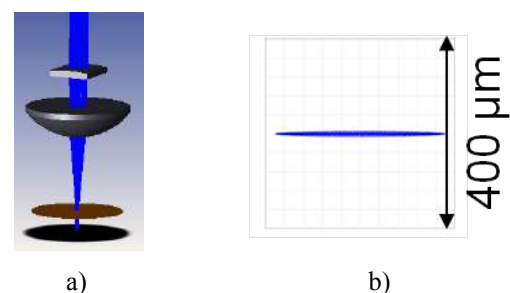
Fig. 14: a) Strahlengang durch eine Zylinderlinse und eine Plankonvexlinse und b) berechnetes Fokussdiagramm des daraus resultierenden Linienfokus.
