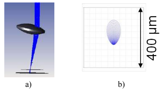
Fig. 12: a) Strahlengang durch außermittig, zur optischen Achse schräg positionierten Bikonvexlinse und b) berechnetes Fokussdiagramm des daraus resultierenden asymmetrischen Fokus.
